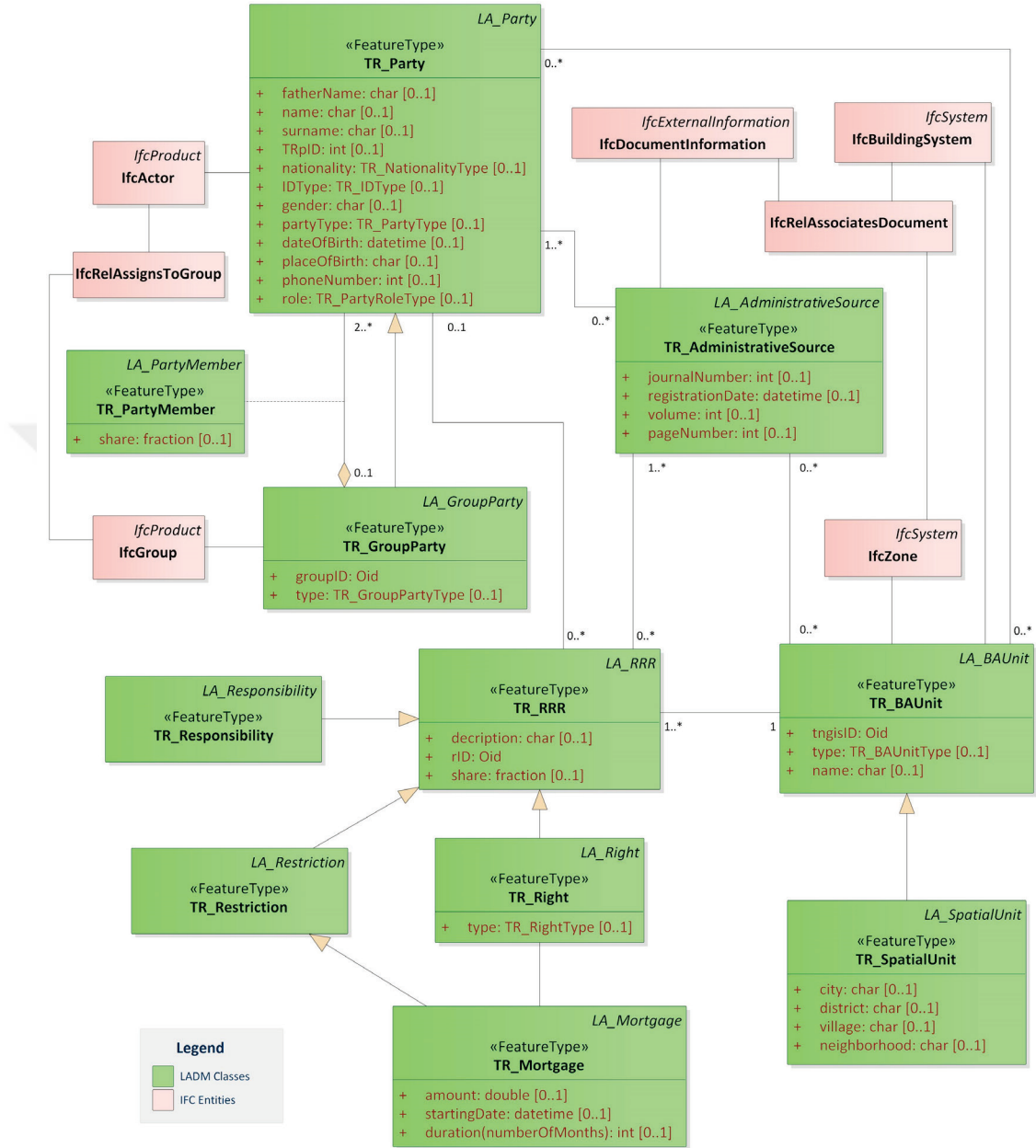
Şekil 3.31 : Geliştirilen modelin LADM standardının Party ve Administrative paketlerine karşılık gelen bölümü.
