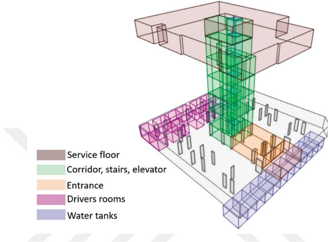
Şekil 3.8 : Ortak mekanların 3B modellenmesi örneği (Alattas ve diğ., 2021).
