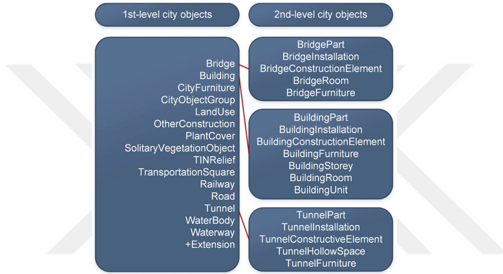
Şekil 2.23 : CityJSON şehir objeleri ve seviyeleri (OGC, 2021a).
